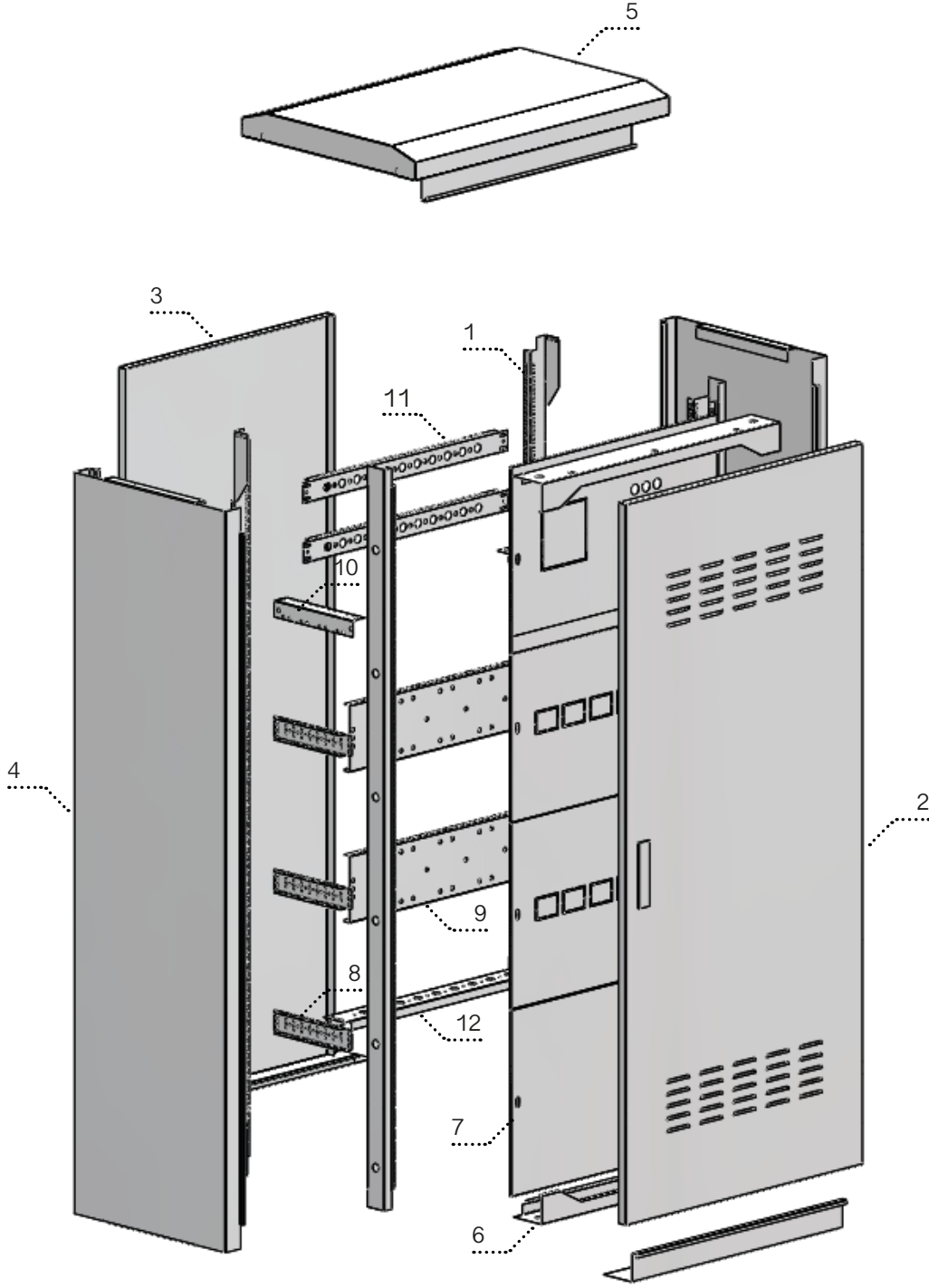
Patlatılmış Görünüm
