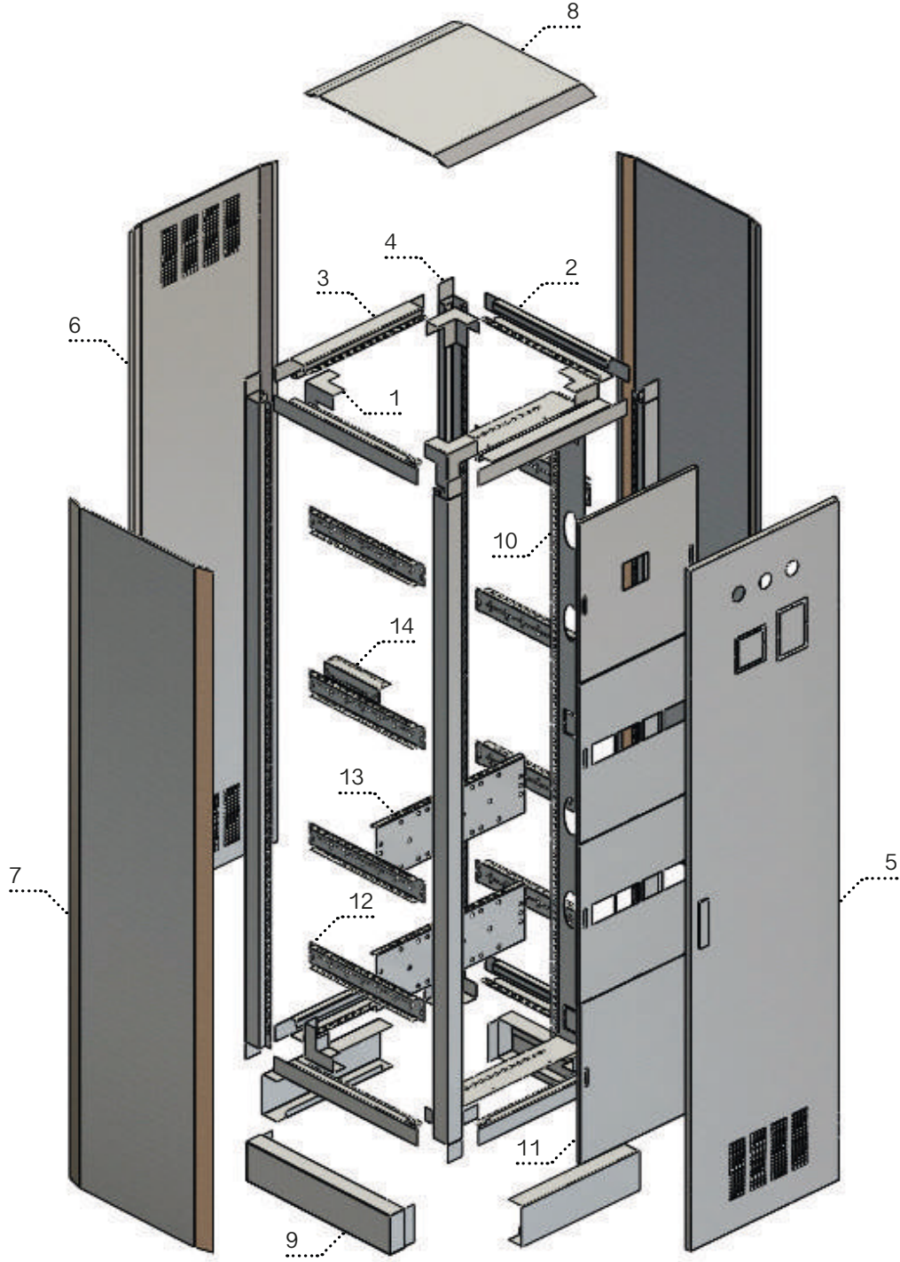
Patlatılmış Görünüm
